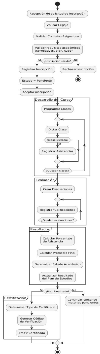
Flujo General del Microservicio Gestión Académica
